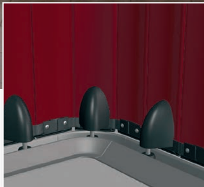
Guidage du tablier par embouts dans le rail bas munis d'une brosse de nettoyage.
